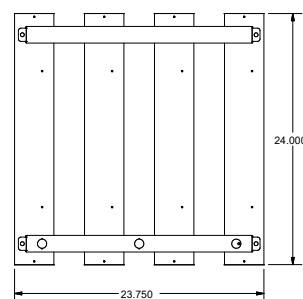
BLSDI 4 Extrémité de guide
