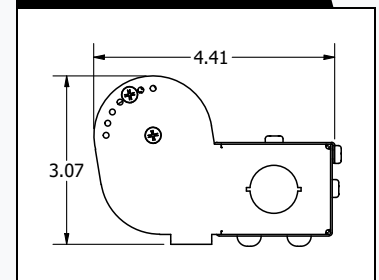
Fin de BLCO
