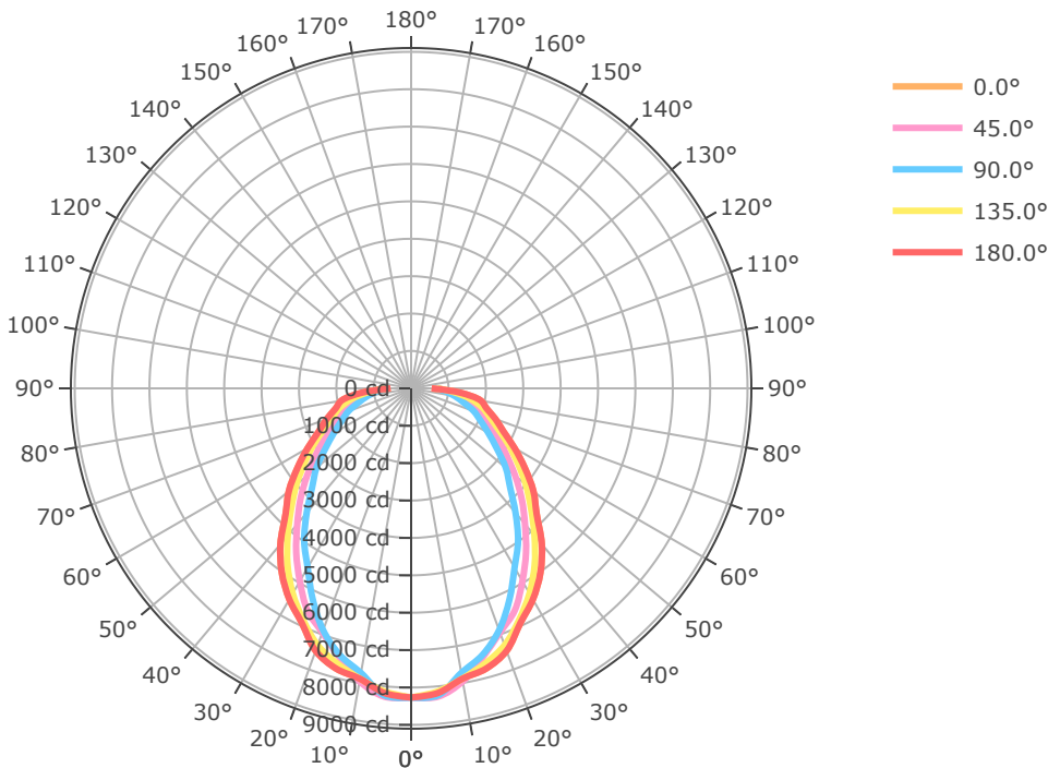
BLHV-2FT-22L-840-L49
