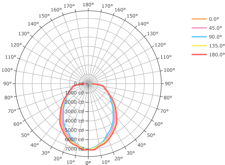
BLHV-4FT-20L-840-L49
