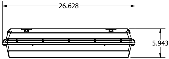
BLHV 2' Side
