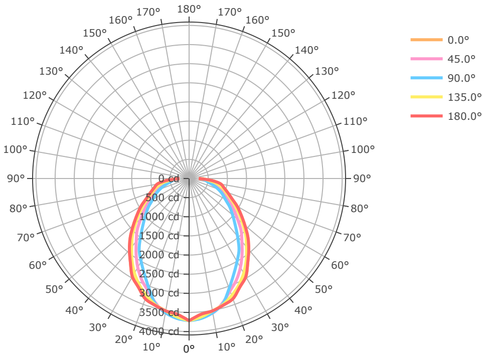
BLHV-2FT-10L-840-L49
