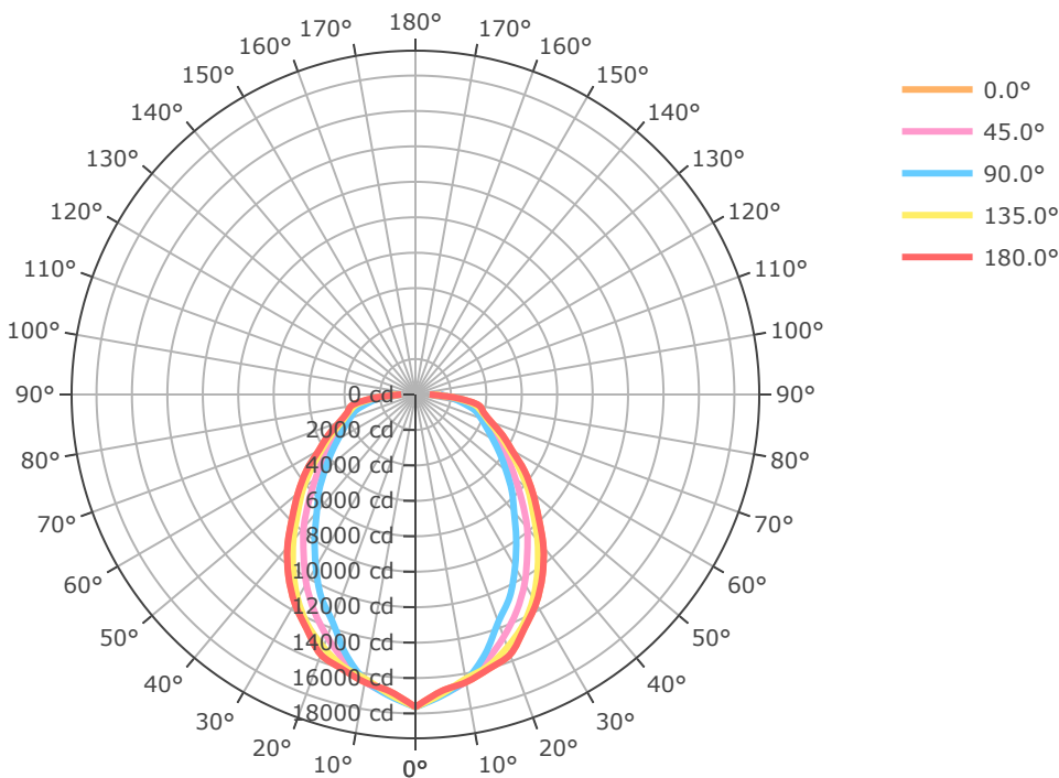
BLHV-4FT-44L-840-L49
