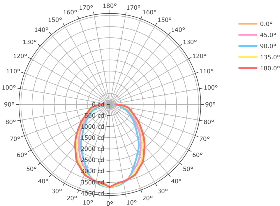
BLHV-2FT-10L-840-L49
