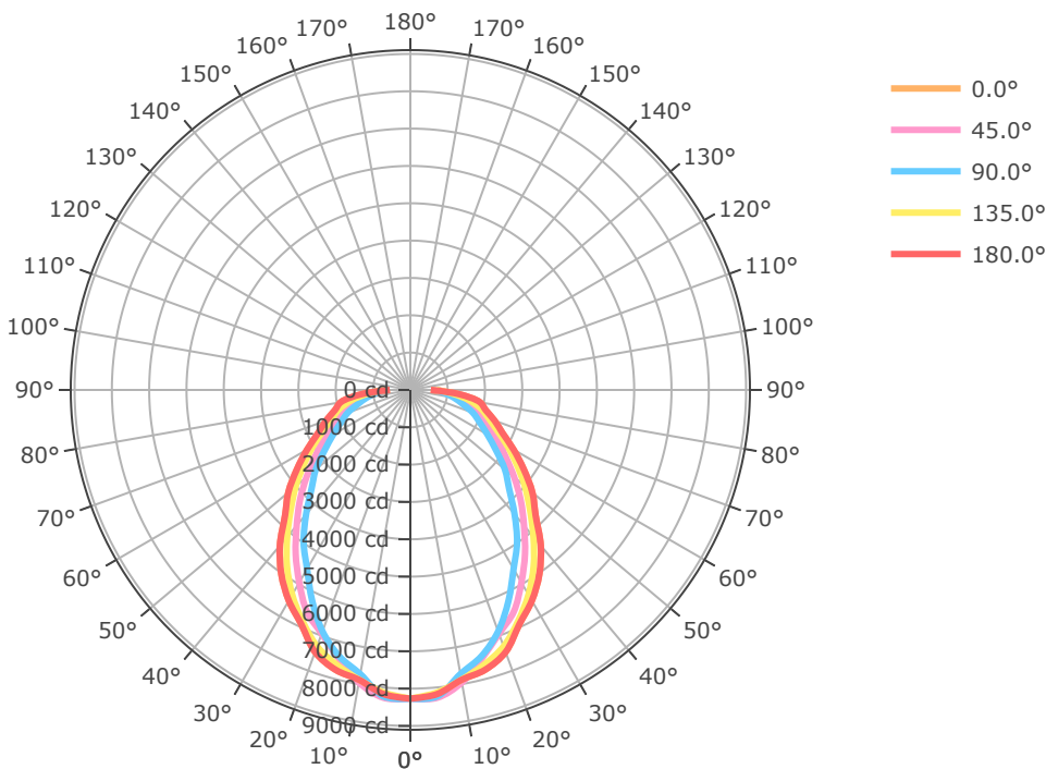
BLHV-2FT-22L-840-L49
