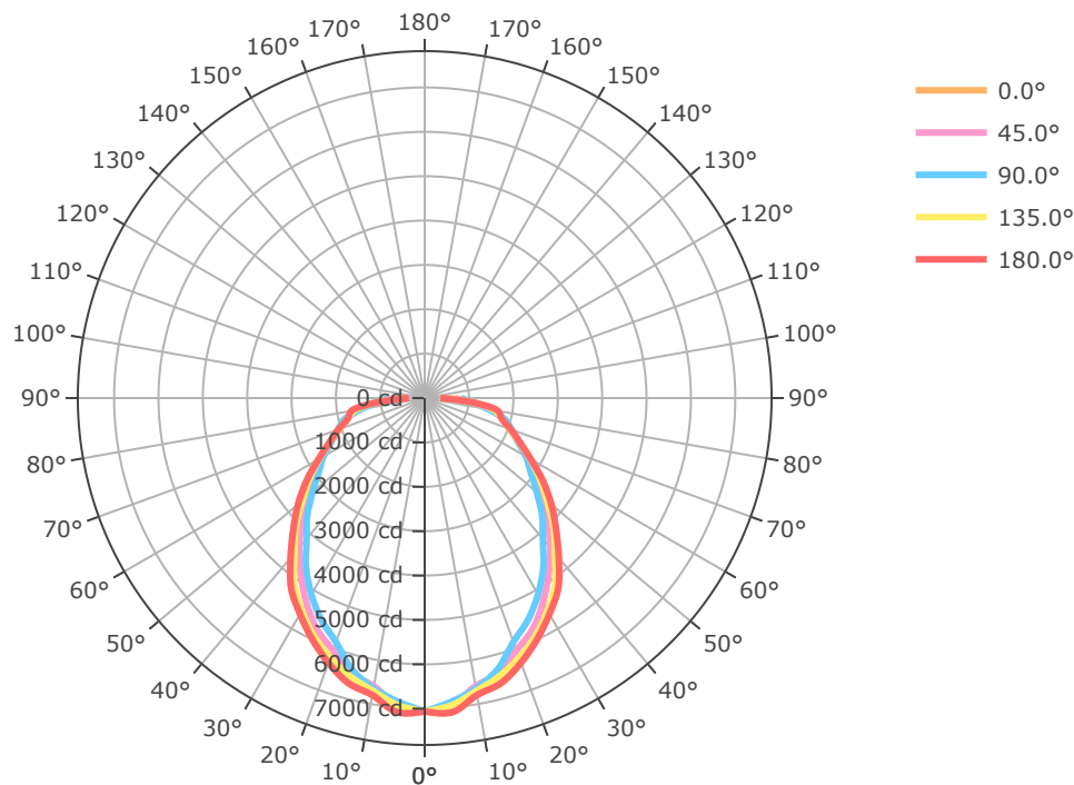
BLHV-4FT-20L-840-L49
