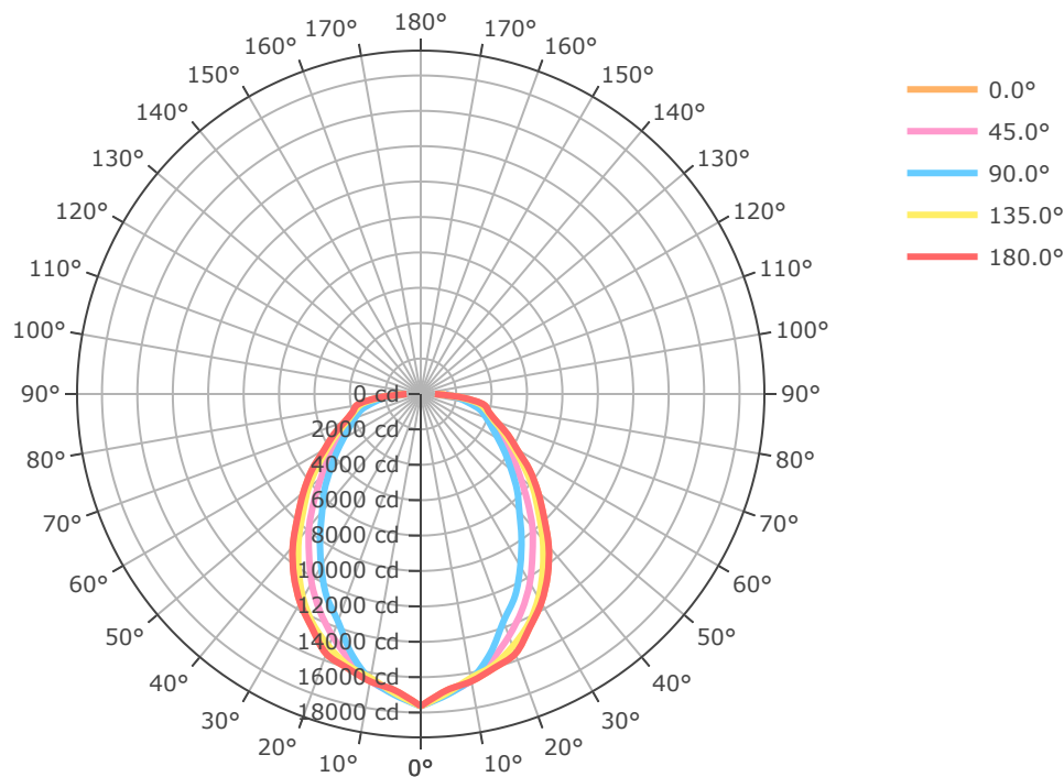
BLHV-4FT-44L-840-L49
