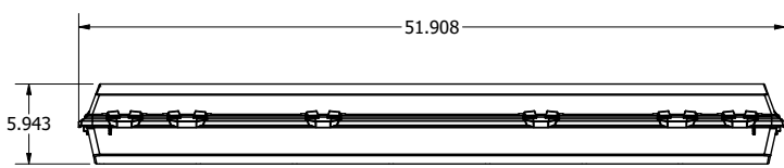
BLHV 4' Side
