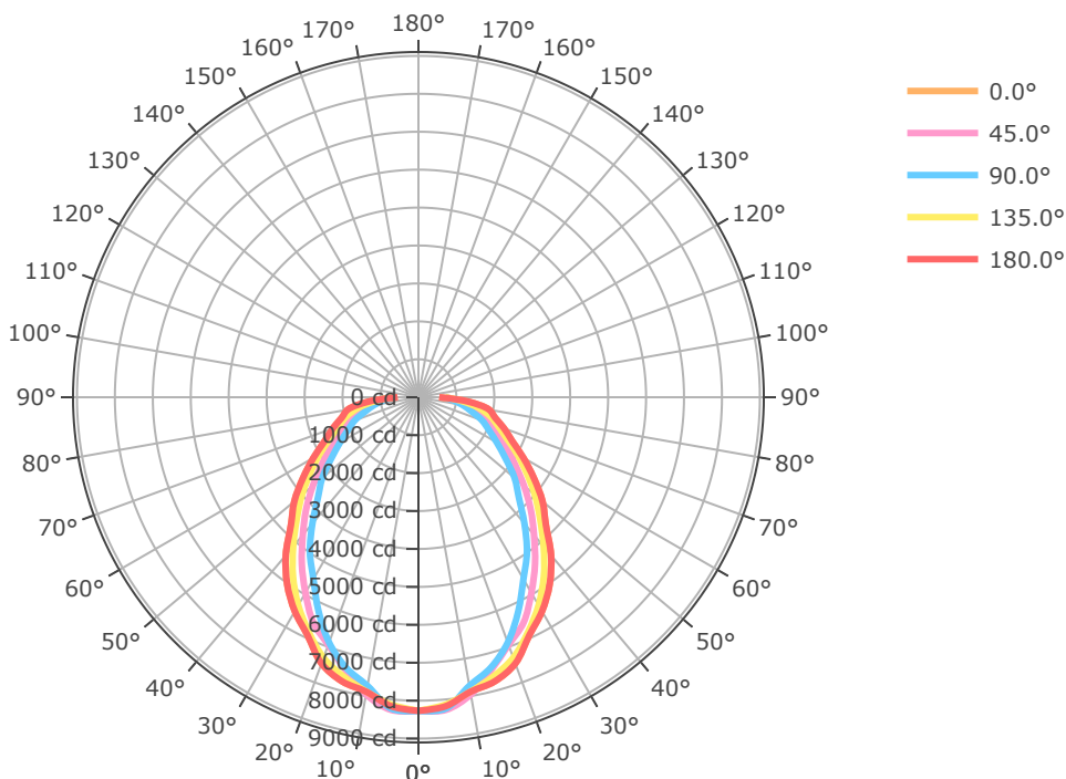
BLHV-2FT-22L-840-L49
