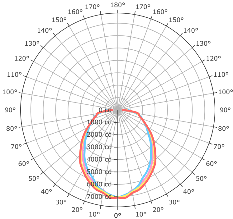
BLHV-4FT-20L-840-L49
