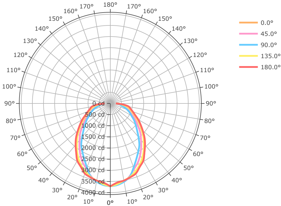
BLHV-2FT-10L-840-L49
