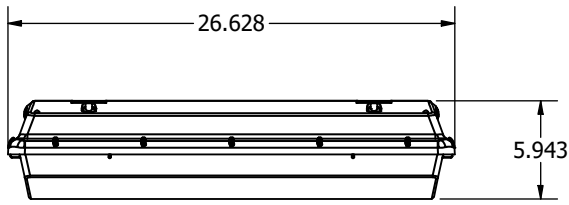
BLHV 2' Side
