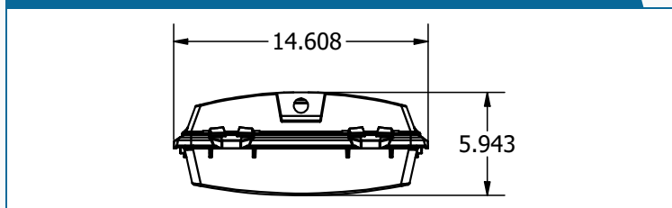
BLHV-H27, extrémité 4'
