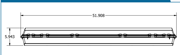
BLHV-H27, côté 4'
