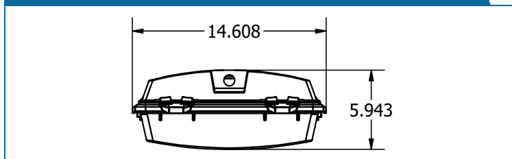
BLHV-H27, extrémité 2'
