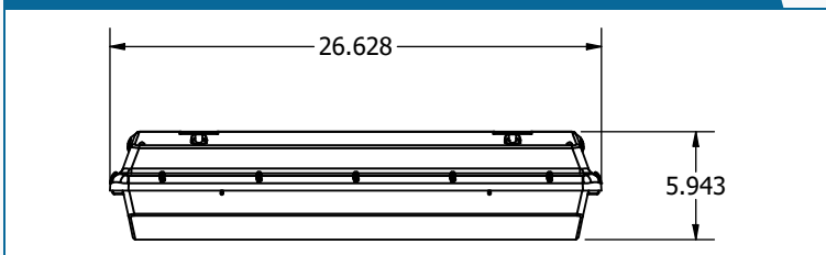
BLHV-H27, côté 2'
