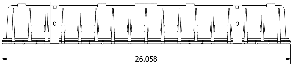
BHZ 2' Dimensiones laterales
