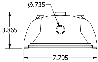
Dimensiones finales
