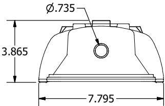
Dimensions de l'extrémité
